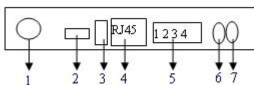
寻呼话筒后面接口草图（从左到右）
