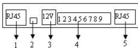
主控机后面接口草图（从左到右）
